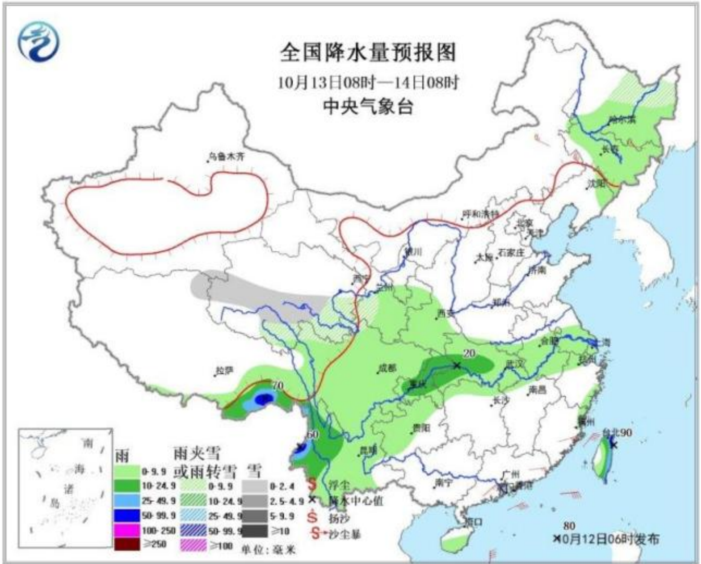
图3 天下降水量预告图(10月14日08时-15日08时)
